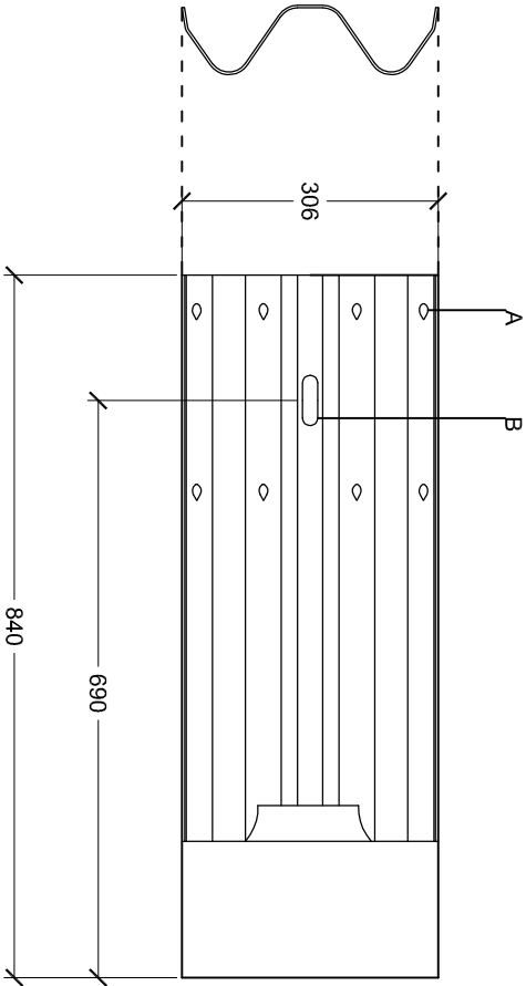
Voorraanzicht drup, niet verkropt
