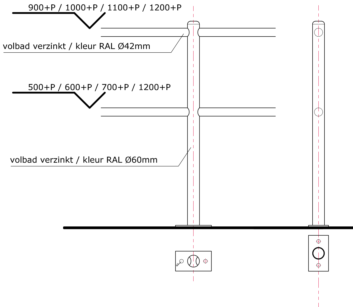
Principe baluster, dubbele uitvoering
